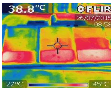
Фиг. 2. Термографска снимка на опитния образец
