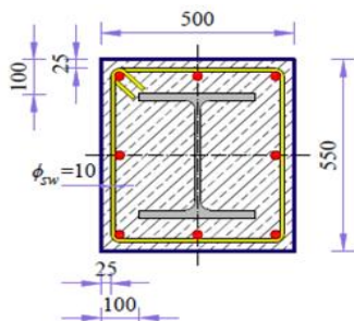
Фиг. 6. Изследвано напречно сечение
