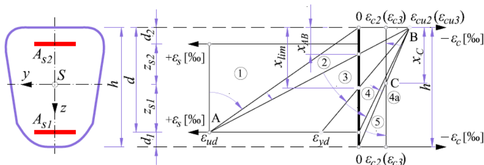
Фиг. 4. Области на напрегнато и деформирано състояние
