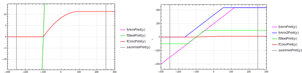
Фиг. 5. Примерни работни диаграми за конкретна стойност на натисквата зона. На бетона (в ляво) и на стоманата (в дясно)
