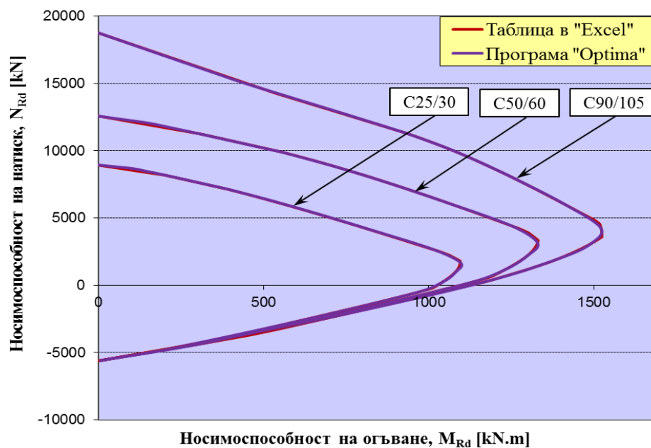
Фиг. 8. Сравнение на криви на носеща способност между програмния алгоритъм и ръчни изчисления
