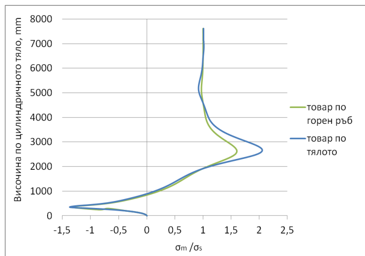
в) GNA – с отчитане на големи премествания на елементите и еластичен материал Фигура 5. Отношение на напреженията \sigma_m/\sigma_s в черупка с несъвършенства
