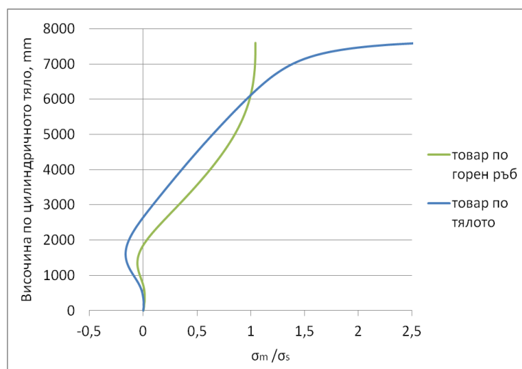
б) MNA - нелинеен материал и малки премествания
